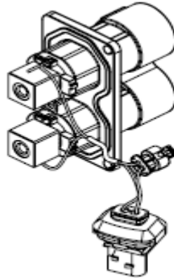
Rys. 2 - Widok złącza prostego – 2 warianty złącza
