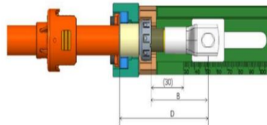
Rys. 1 – Widok wiązki przed procesem założeniu i obkurczenia rurki termokurczliwej HD1400 – 95mm 2 , 120mm 2 , 150mm 2
