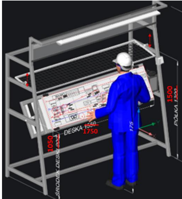
Rys. 1 – Rysunek poglądowy konstrukcji obrotowej
