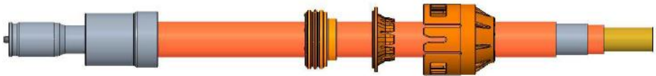
Rys. 1 – Widok wiązki przed procesem domyknięcia gumy i osłony na przewodzie – złącze HD1400 – 95mm 2 , 120mm 2 , 150mm 2
