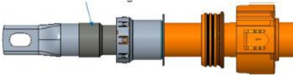
Rys. 4 – Widok wiązki przed procesem domyknięcia gumy i osłony na przewodzie – złącze IPT HD – 120mm 2 , 150mm 2
