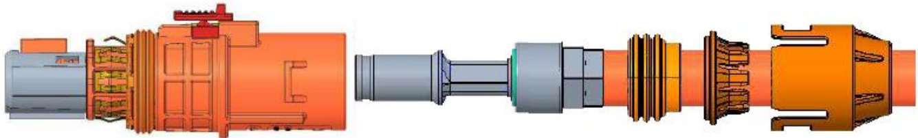
Rys. 2 – Widok wiązki przed procesem domyknięcia gumy i osłony na przewodzie – złącze HD1000 – 50mm 2
