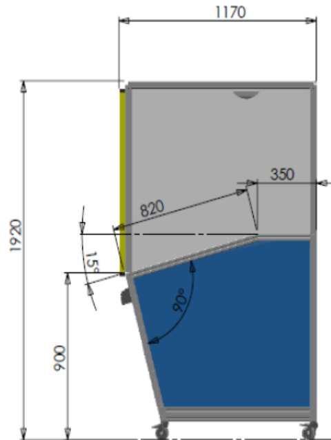
Rys. 1 – Graficzne przedstawienie wymaganej wymiarowości stołu testującego
