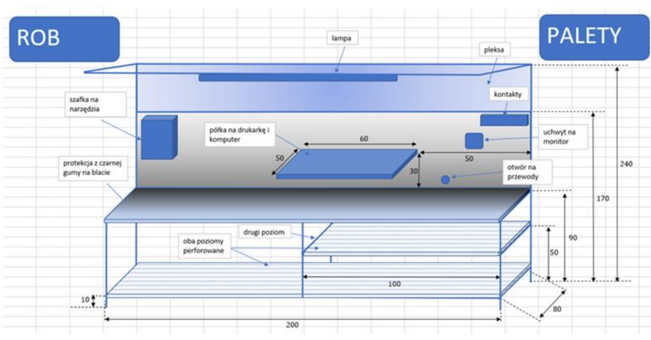
Rys. 1 – Przykładowy widok stanowiska do pakowania
